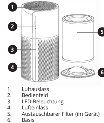
Bedienfeld
