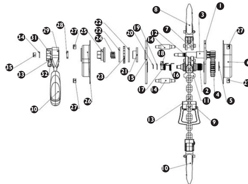
IX. SCHÉMA D'ENSEMBLE DE LA MACHINE
