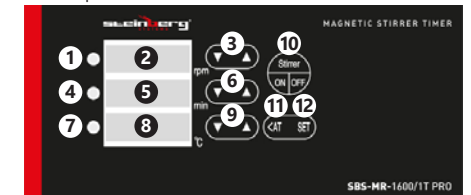
SBS-MR-1600/1T PRO
