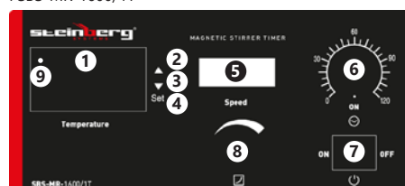
Panel de control de los modelos SBS-MR-1600/6 i SBS-MR-1600/1T
