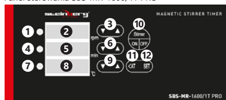
Panel sterowania SBS-MR-1600/1T PRO
